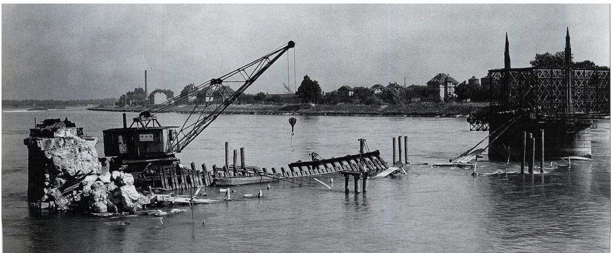
Abb. 6: Am 2. September 1940 waren die in den Rhein gestürzten Brückenteile der Kehler Brücke zum Teil für den anstehenden Wiederaufbau beiseite geräumt. Aufnahme: SLG, Reinhard Schulz, in: Scharf, 2003 (wie Anm. 33), S. 67. In diesem Zustand konnte die Brücke einen Monat später nicht benutzt werden.
